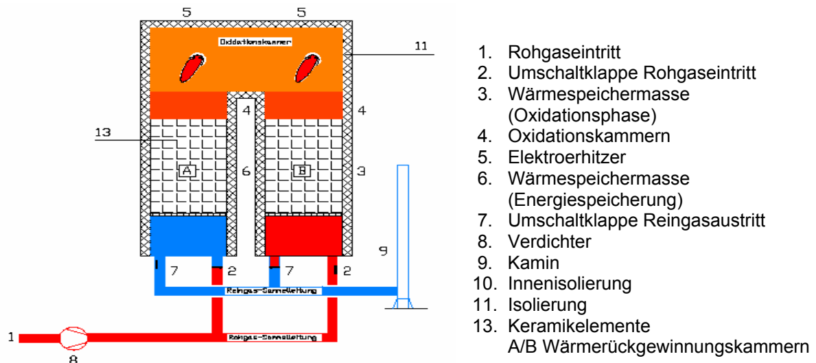
Abbildung. 15: Verfahrensschema der Nachverbrennung im DEPOTHERM ® -Reaktor (Druckbetrieb) [UMAT 2005]
