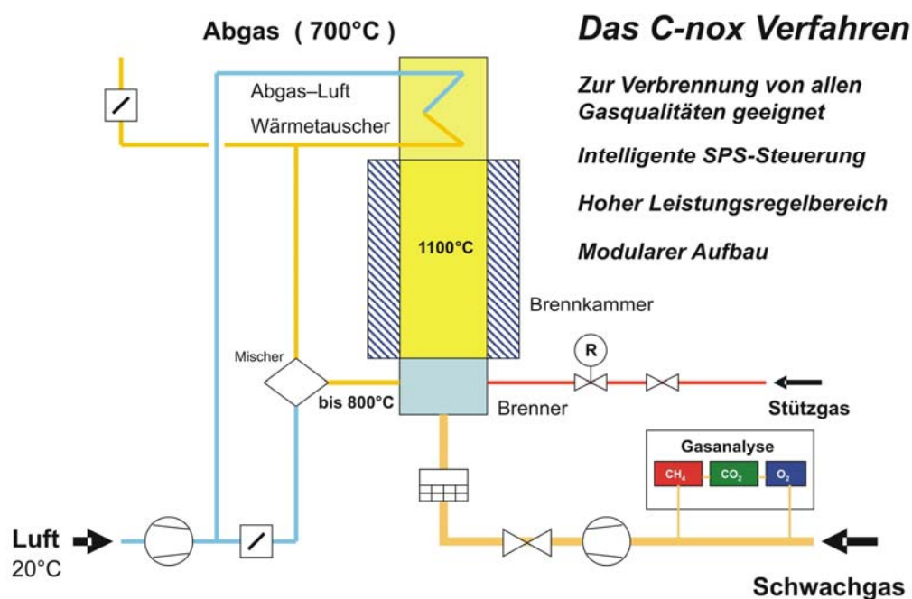
Abbildung. 13: Funktionsschema der C-nox Schwachgasfackel [HEGEMANN UND KÜGLER 2007]
